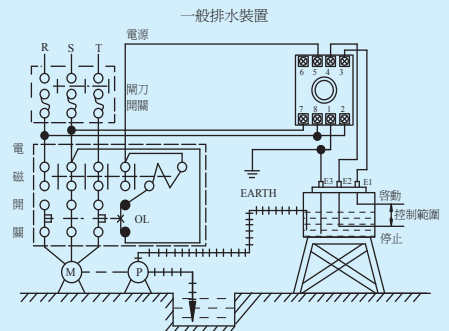
General Drainage Running 一般排水裝置
