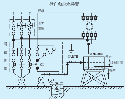
General Water-Supply Running 一般自動給水裝置
